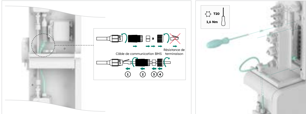
Entre les batteries / Entre l'onduleur et la première batterie
