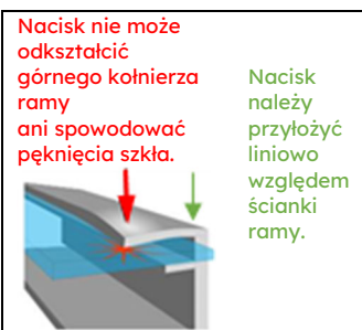
Rysunek 1a: Miejsca przyłożenia
