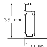
RAHMENPROFIL VON DER SEITE
