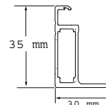
BOCZNY PROFIL RAMY
