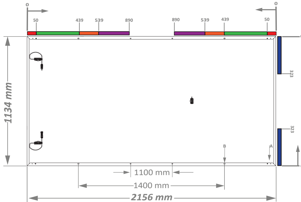
A - Trous pour mise à la terre (4X @ 4,2mm) B - Trous de montage (8X 9mm (W) x 14mm (L), R4,5mm)
