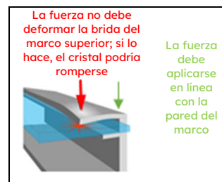
Figura 1a: Ubicaciones de fuerza de abrazaderas
