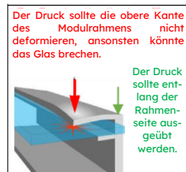
Abbildung 1a: Druck auf die Klemmenstellen
