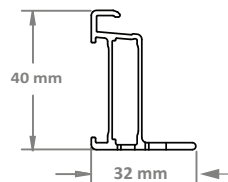
PROFIEL VAN ZIJFRAME
