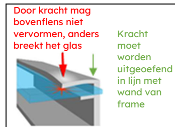
Afbeelding 1a: Locaties voor klemkracht
