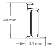
PROFIEL VAN EINDFRAME
