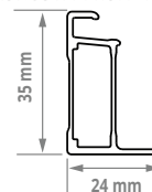
KOŃCOWY PROFIL RAMY
