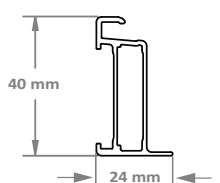
ENDE DES RAHMENPROFILS
