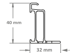
PRAHMENPROFIL VON DER SEITE
